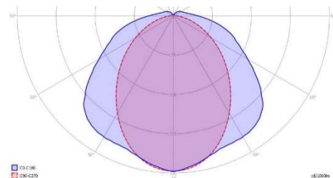
SVĚTLNÁ CHARAKTERISTIKA DISTRIBUTION OF LUMINOUS INTENSITY
